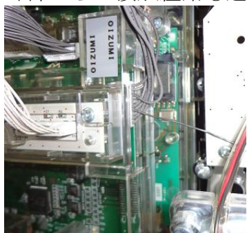
サブ基板
